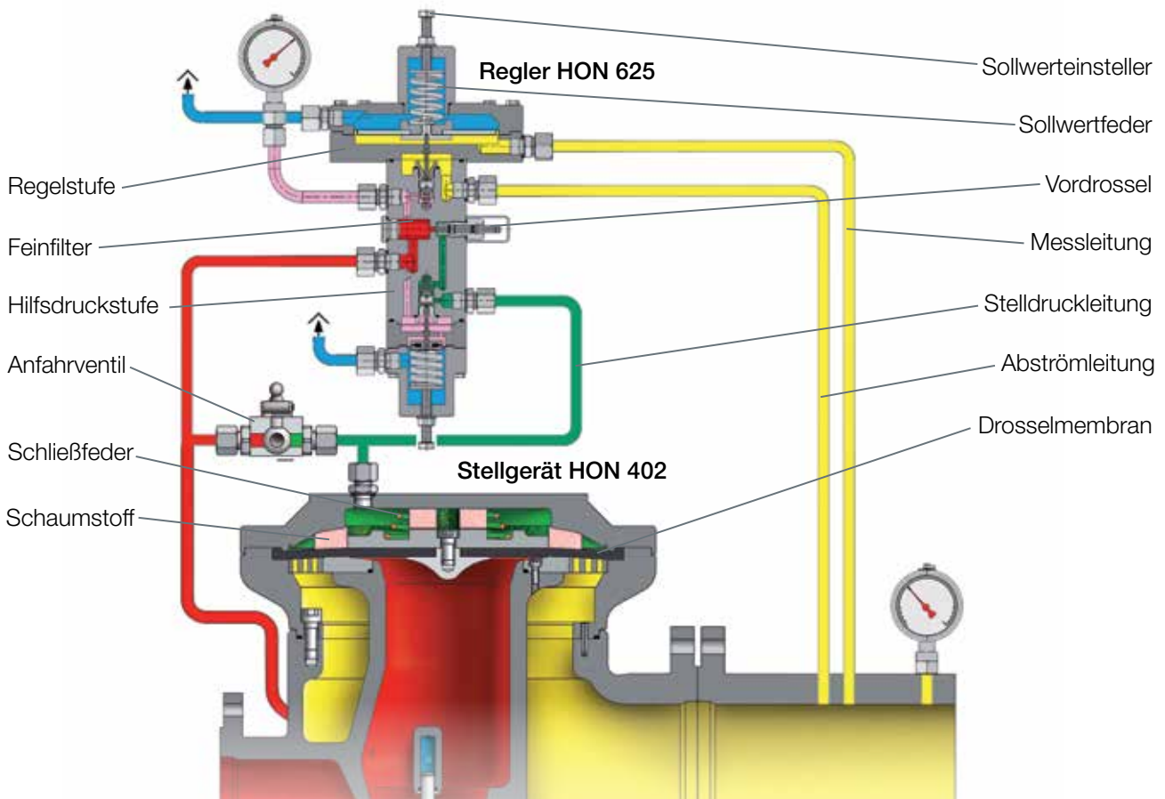
Fließbild des Gas-Druckregelgerätes HON 402 mit HON 625
